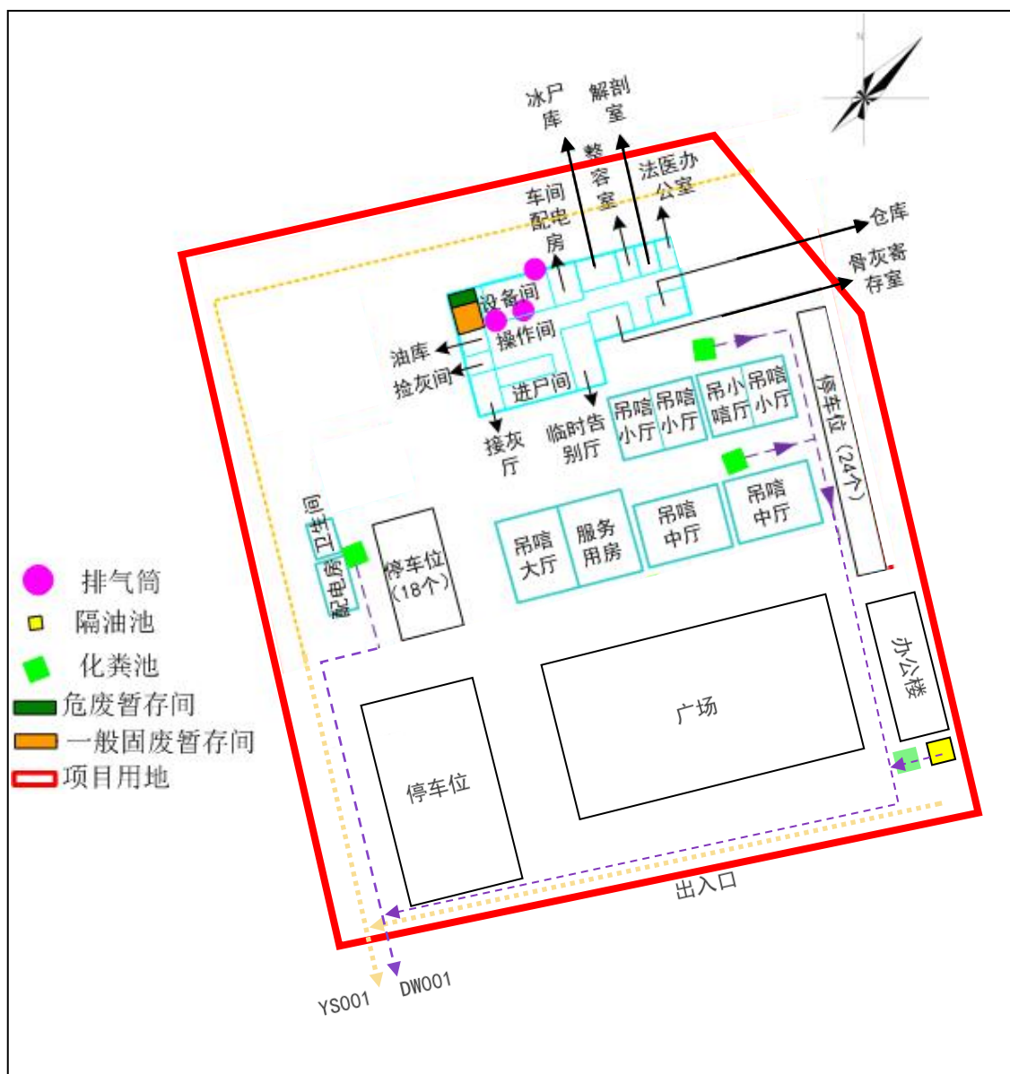
附图 3 项目平面布置图及雨污管网图
